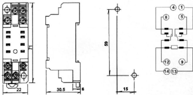
外型圖 開孔尺寸 接線圖 (OUTLINE) (DRILLING PLAN) (WIRING DIAGRAMS)
